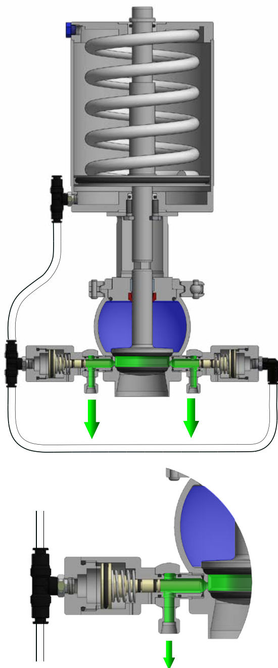
Fig. 1 VALVOLA CHIUSA
