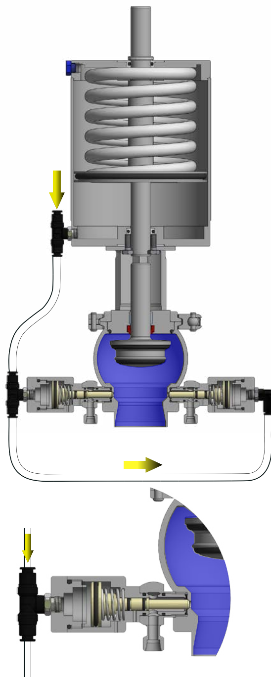
Fig. 2 VALVOLA APERTA
